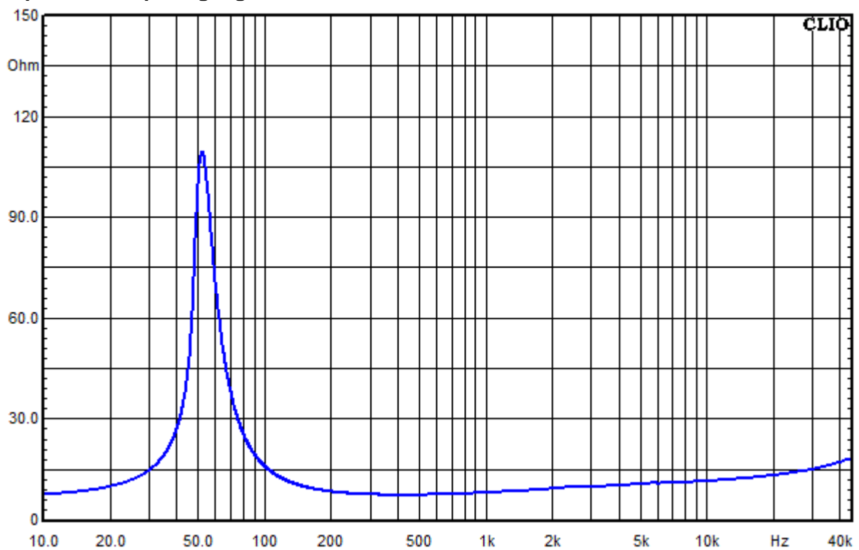
Abbildung 4: Wavecor WF120CU08-Impedanzverlauf
